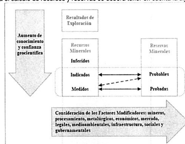
Figura 4. Relación general entre los resultados de exploración, recursos minerales y reservas minerales.
