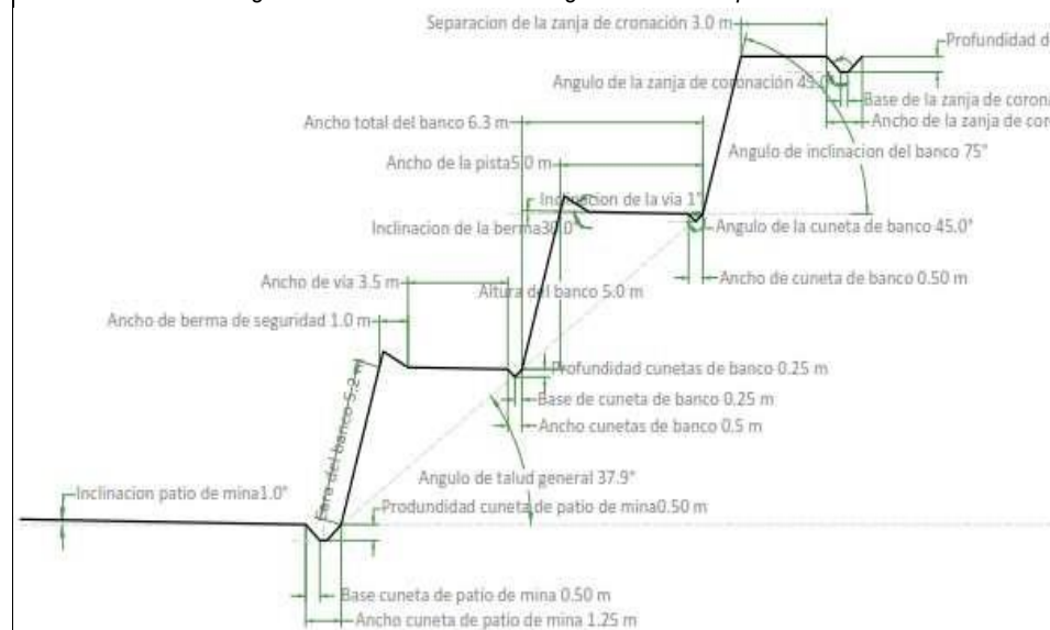
Figura 4.39 Dimensionamiento general de la explotación
