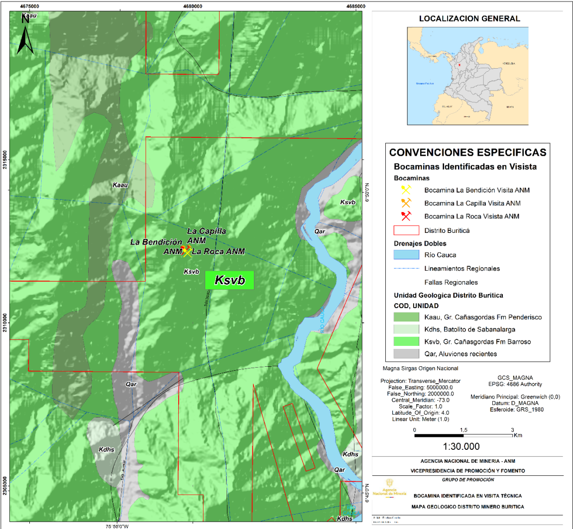
Figura 5. Mapa geológico. Fuente: Elaboración propia con base en el Informe del SGC “Evaluación del potencial mineral para oro en el distrito de Buriticá, departamento de Antioquia”.
